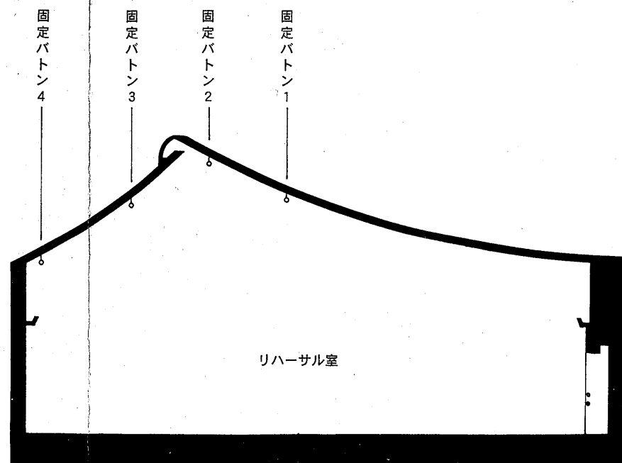
リハーサル室断面図 S=1/100
